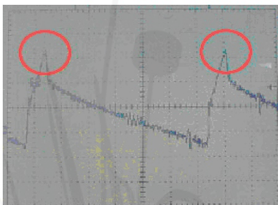
Rövidoldali kivezetés : a kapcsolási impulzusok zajosak
